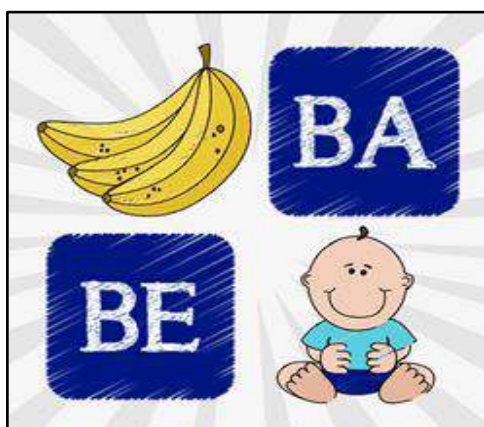
Figura 2: Aplicativo Silabando
